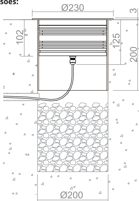
Dimensões em mm. Nicho: Ø200mm.
