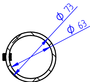
Seção A-A
