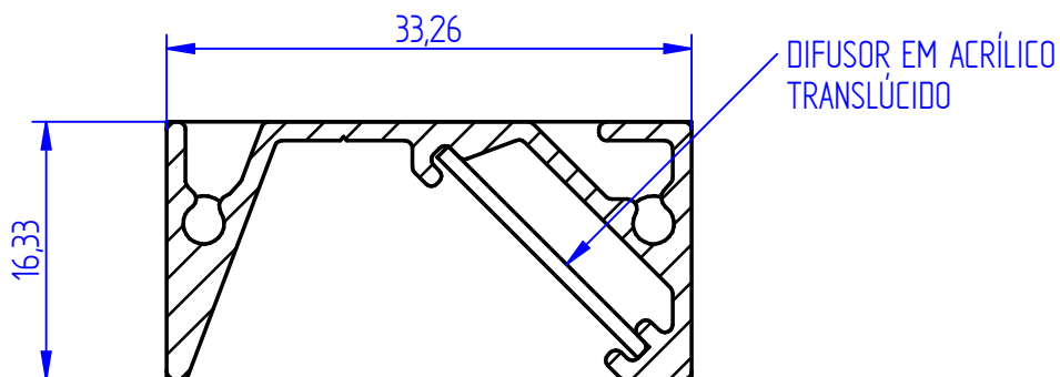
Seção A-A
